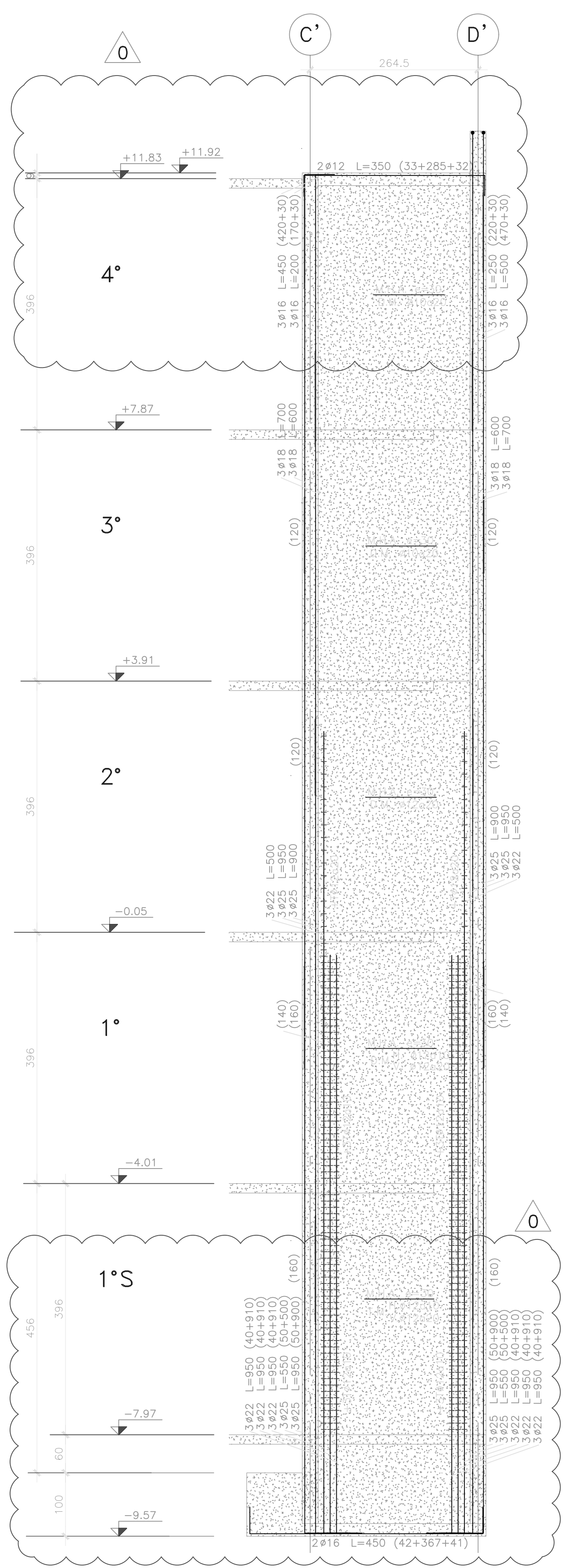
ELEVACION EJE 1' ESCALA 1:50
